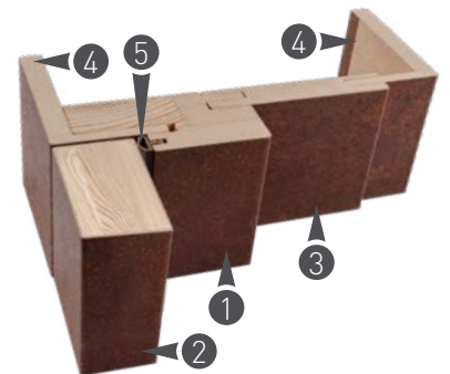
РОЗРІЗ ЩИТОВОГО ДВЕРНОГО БЛОКА
